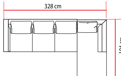
Modulacija STL
