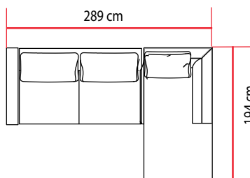
Modulacija SDL
