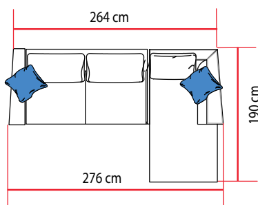
Modulacija SDL
